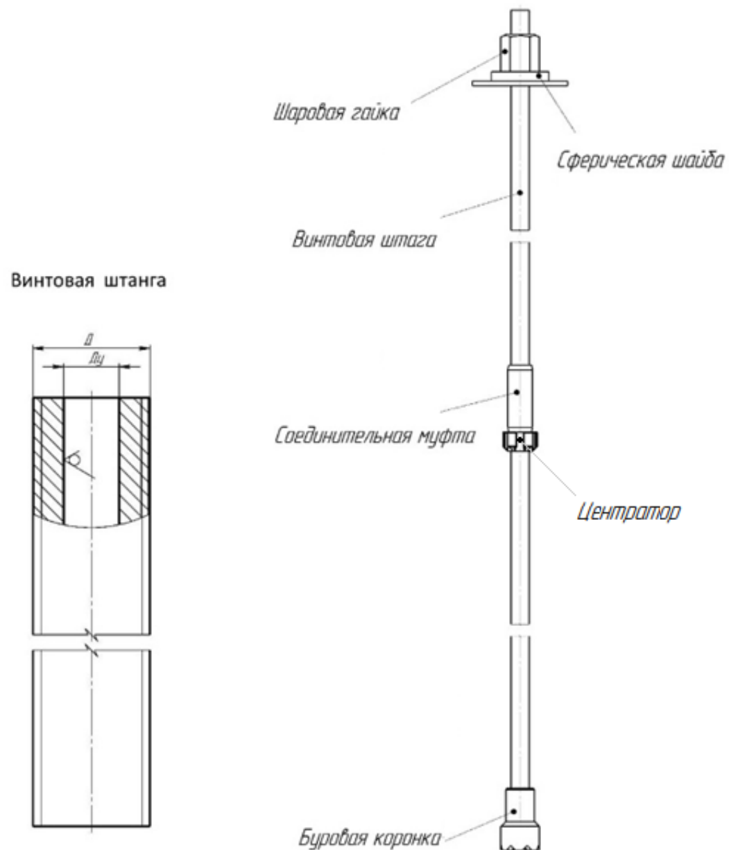
АНКЕР ГРУНТОВЫЙ "АКБС" общий вид:
